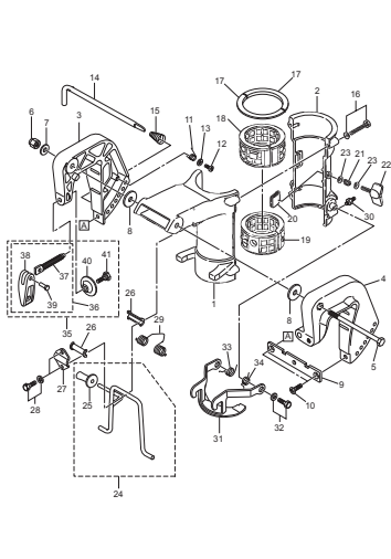
Fig. 8 BRACKET • REVERSE LOCK ARM ブラケット・リバースロックアーム
