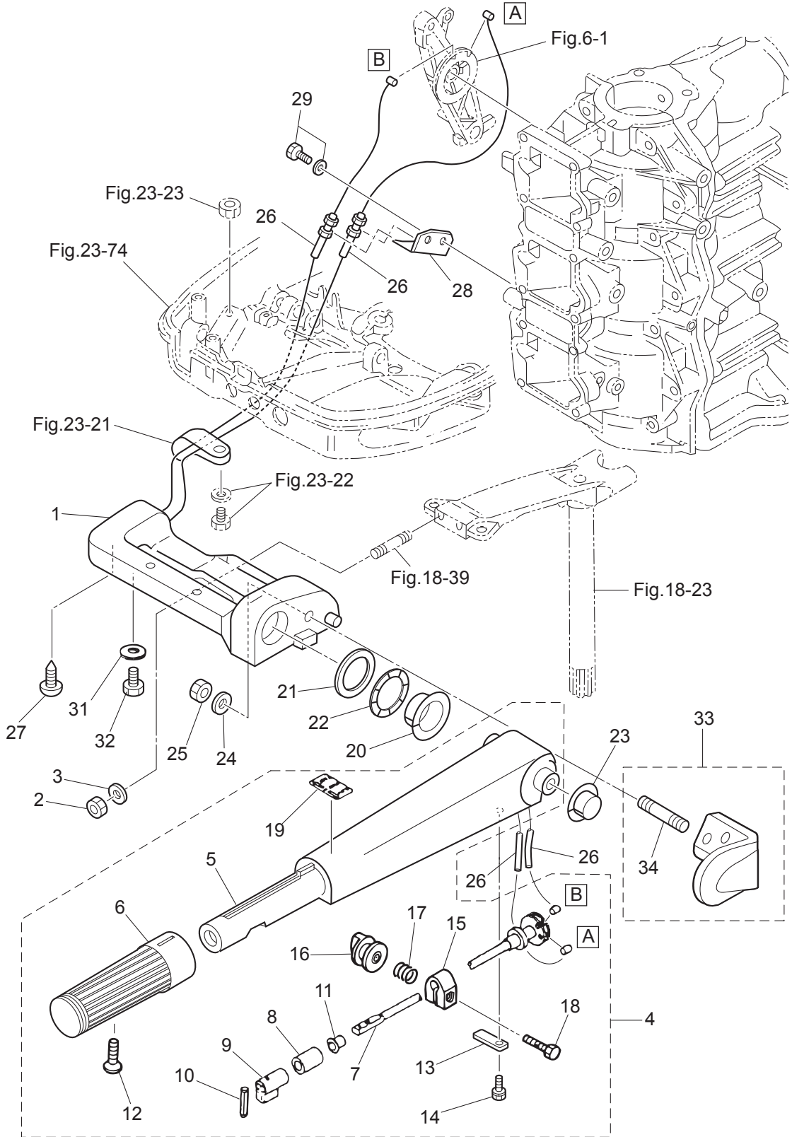
TILLER HANDLE (F TYPE) ティラハンドル (F タイプ)
