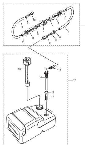
Fig. 28 ACCESSORIES アクセサリー
