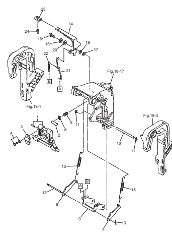
Fig.19 MANUAL TILT マニュアルチルト
